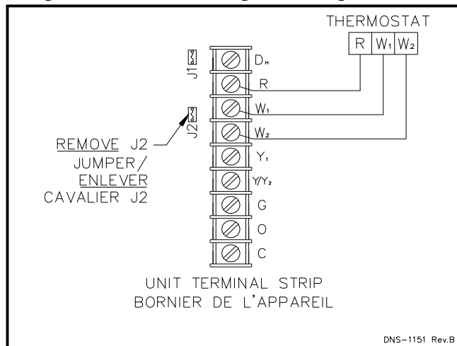
Figure 5 : Thermostat 2 stages, chauffage seulement
