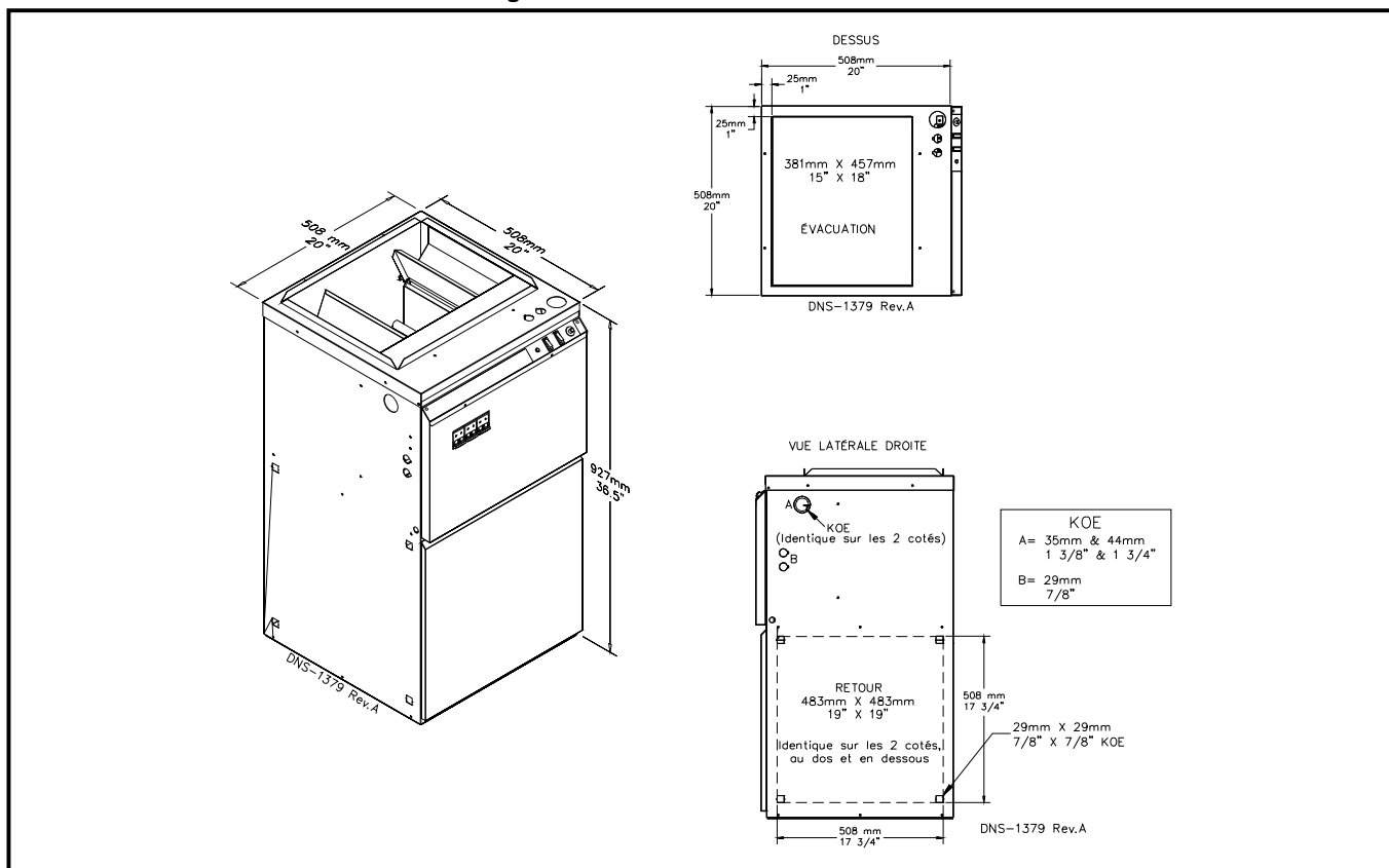
Figure 14 : Dimensions de la fournaise
