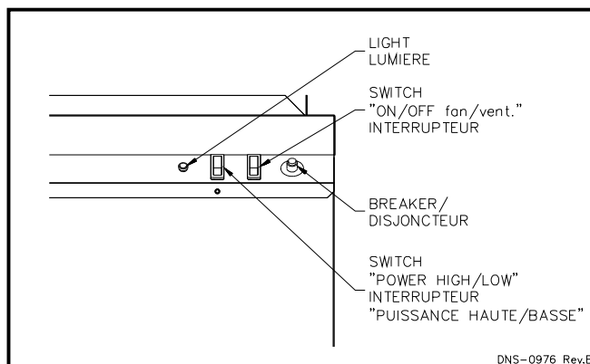
Figure 13 : Commandes manuelles sur la fournaise
